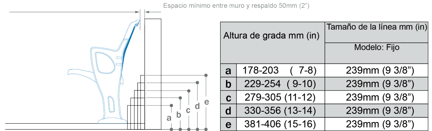
Tamaño de la línea: Distancia tomada del barreno delantero de la pata a la grada
